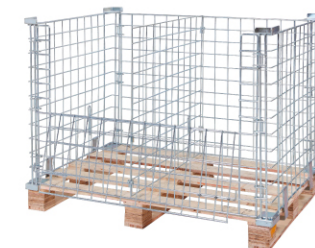
YRD-P1 L×W×H: 1200×1000×860 (mm)
